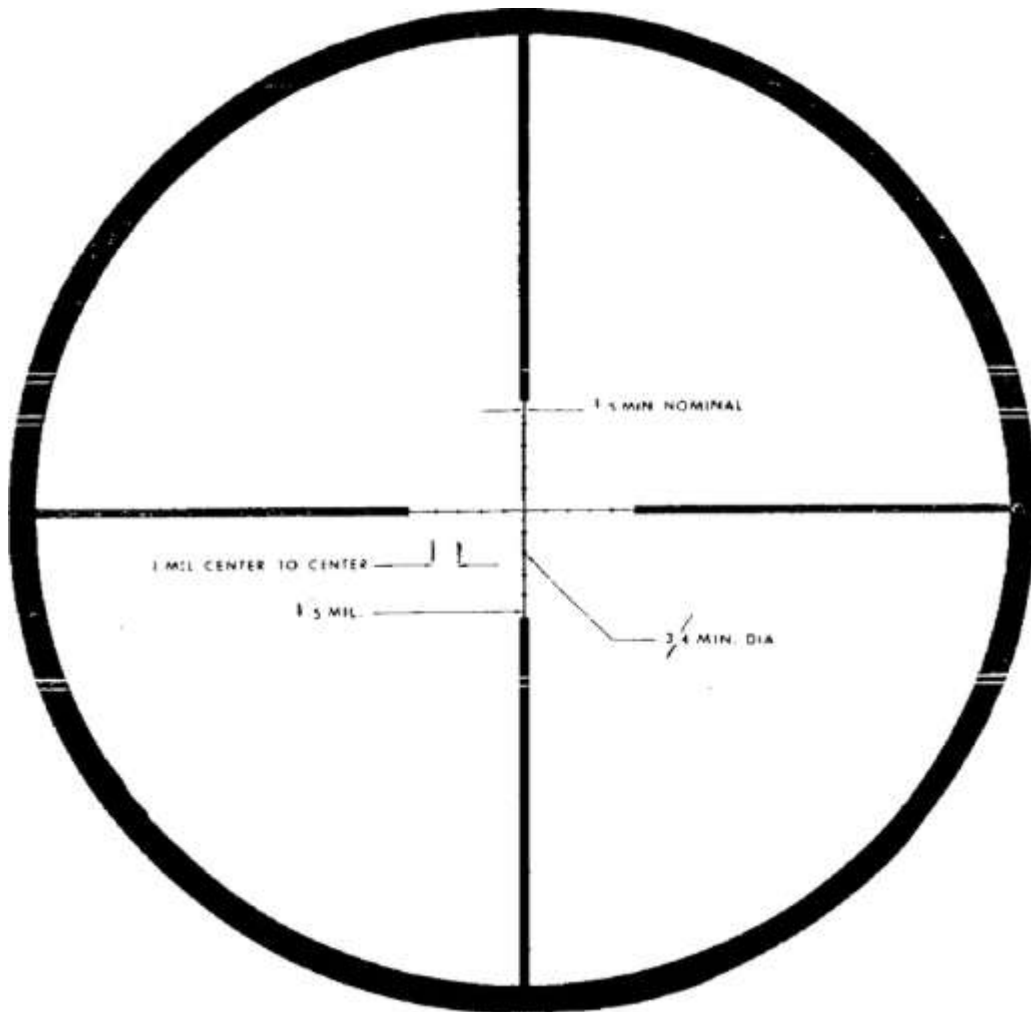
3/4 Min. Mil Dot Reticle Fig. #3
