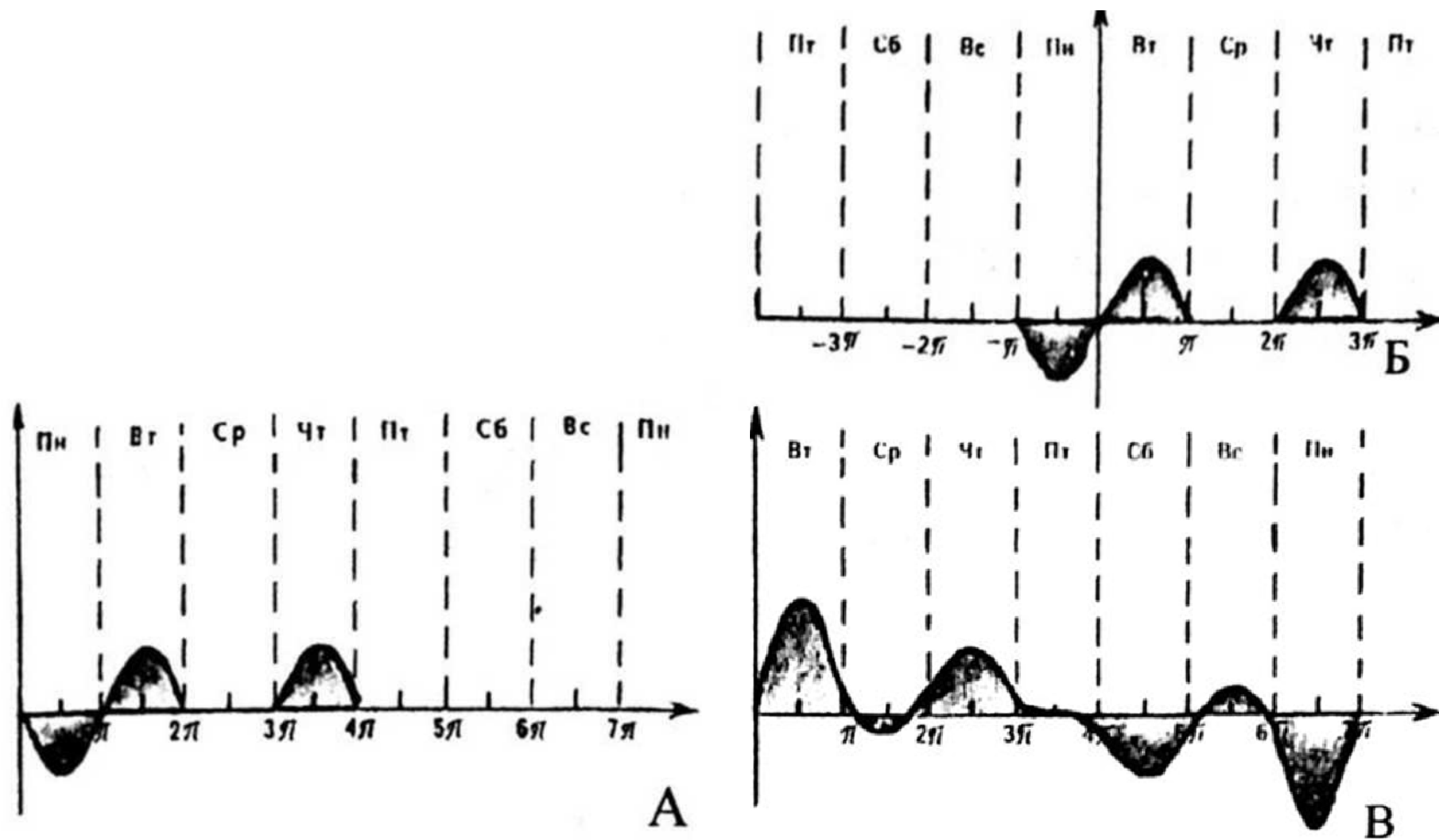
Рис. 22. Функции А.А. Мальцева.
